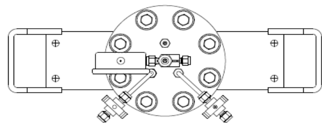
1.5～3Lタイプ(ボール or ストップ弁)
